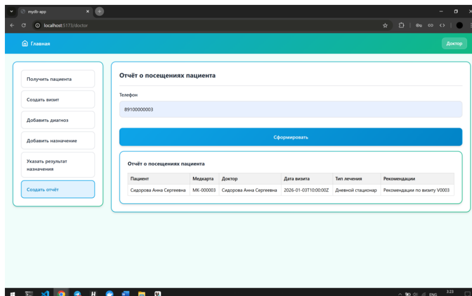
Рисунок 3.2.3.7 - Экранная форма запроса «ОтчётПоВизитамПациента»
