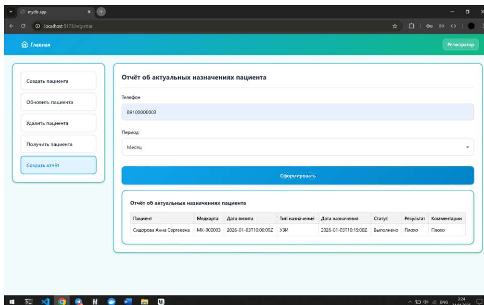
Рисунок 3.2.3.9 - Экранная форма запроса
