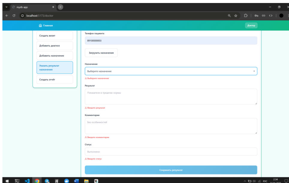
Рисунок 3.2.2.13 - Экранная форма «Указать результат назначения»
