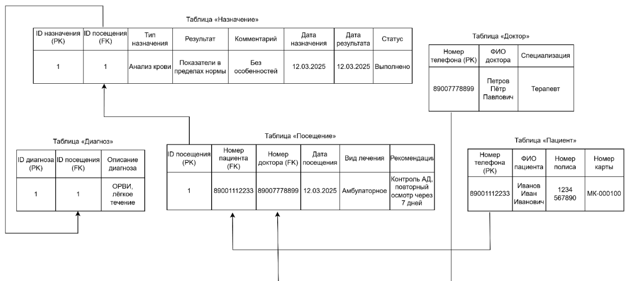
Рисунок 2.2.6.1 - Схема отношений для таблиц «Пациент», «Доктор», «Диагноз», «Посещение», «Назначение»
