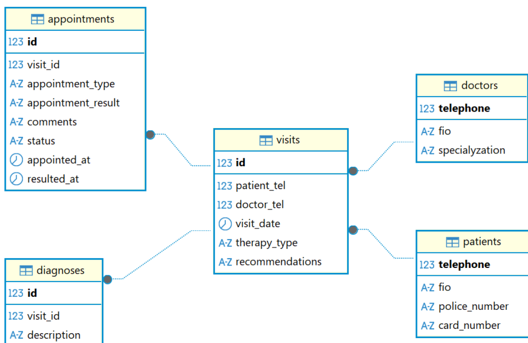
Рисунок 3.2.1.8 - Схема отношений в СУБД PostgreSQL
